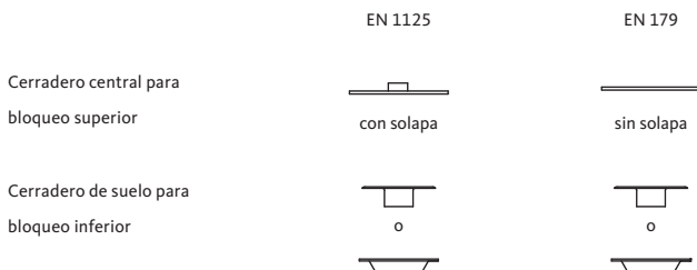
Fig. 3: contornos de cerraderos aprobados
