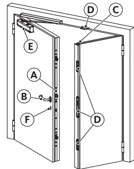
Abb. 1: Verschlusskomponenten
