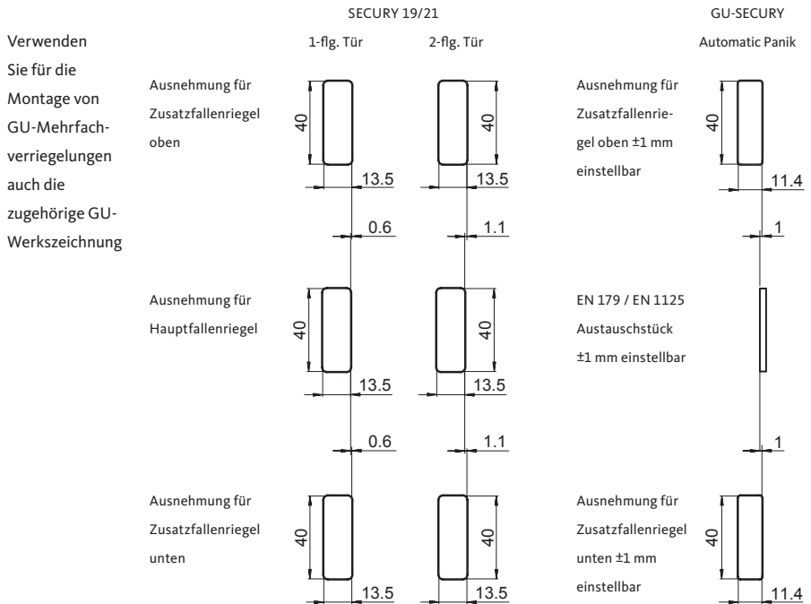
Abb. 4: zulässige Schließblechkonturen
