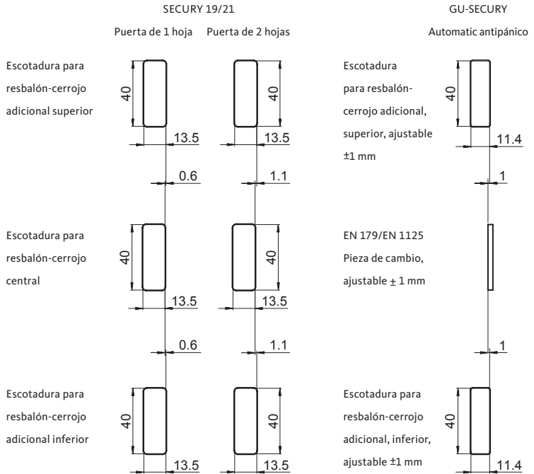
Fig. 4: contornos de cerraderos aprobados
